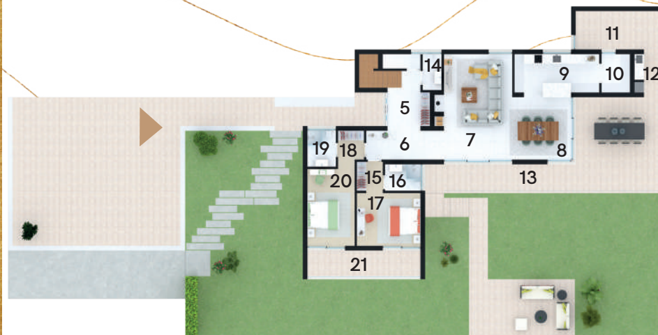
Planta Piso 1
